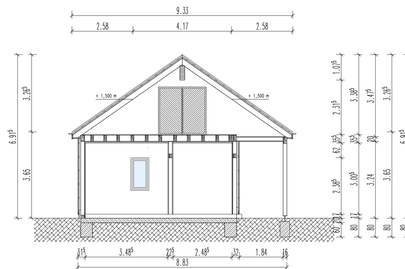
SCHNITT B-B
