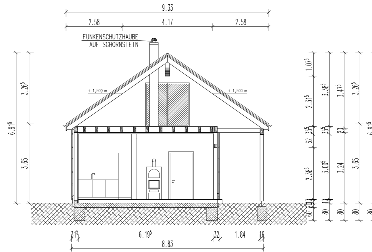
SCHNITT A-A
