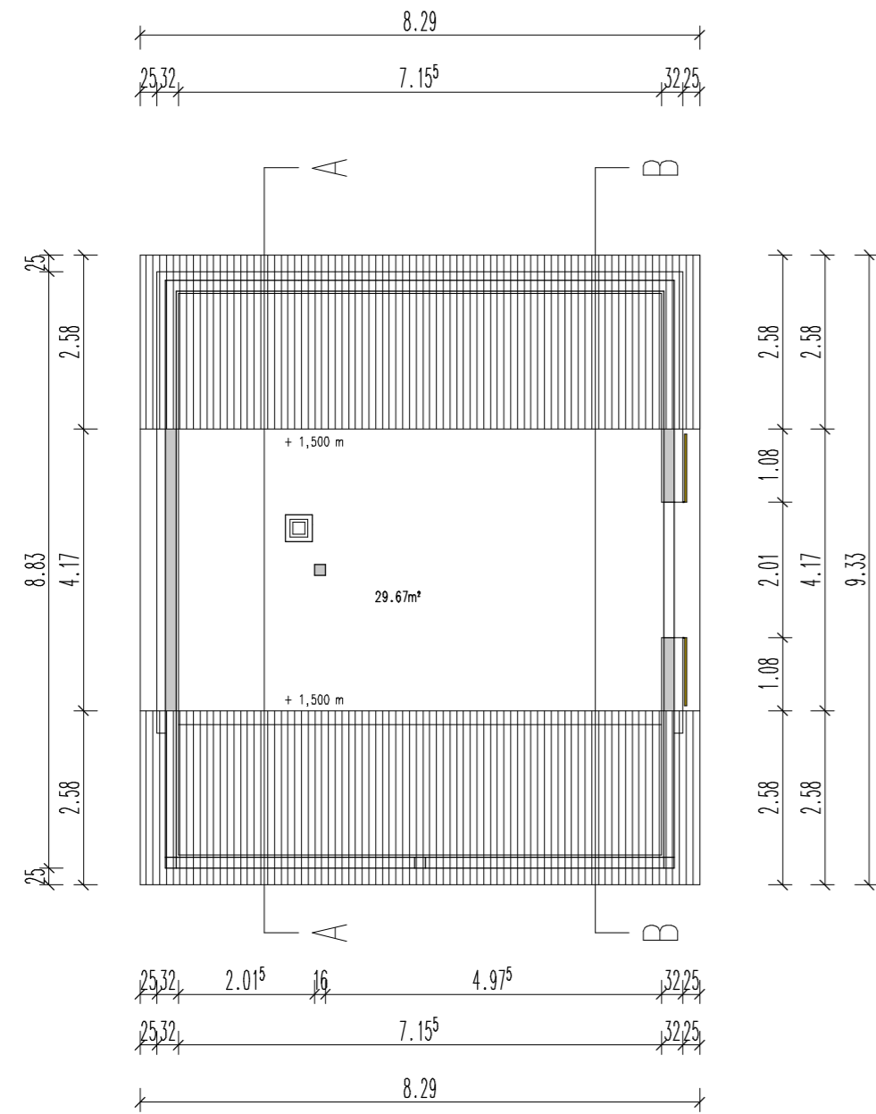
GRUNDRISS DACHGESCHOSS
