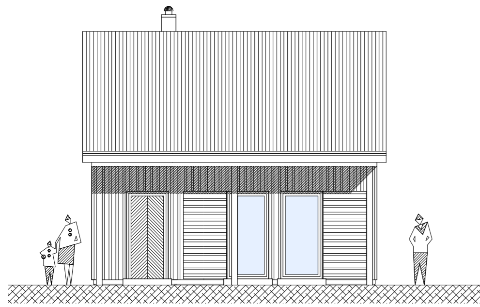
ANSICHT SÜDWESTEN
