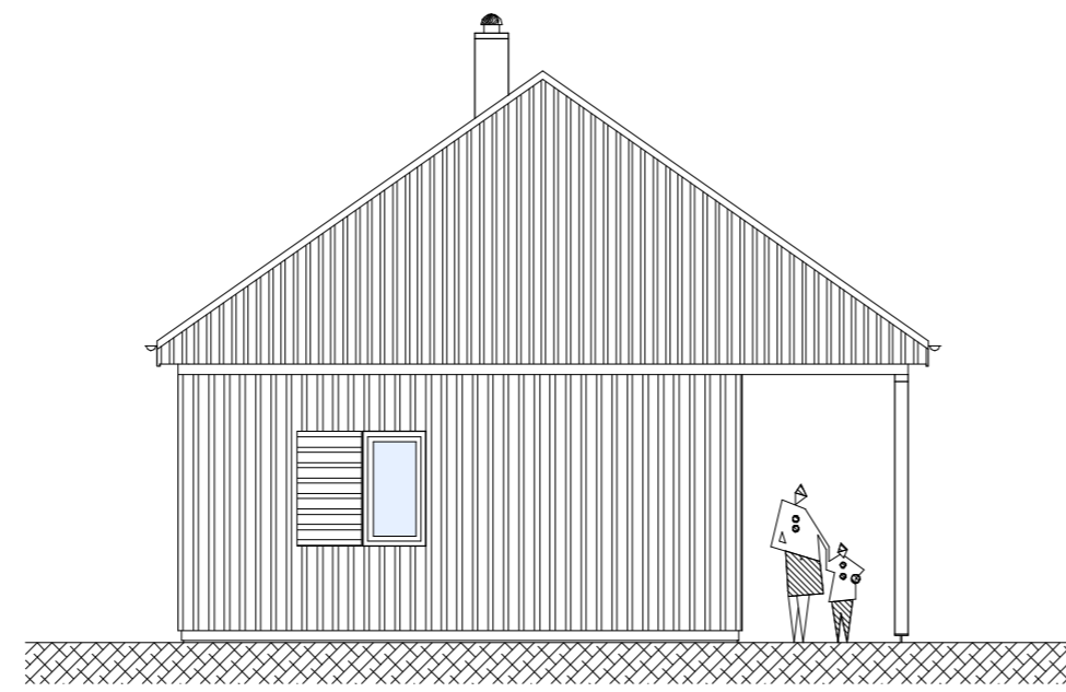
ANSICHT NORDWESTEN
