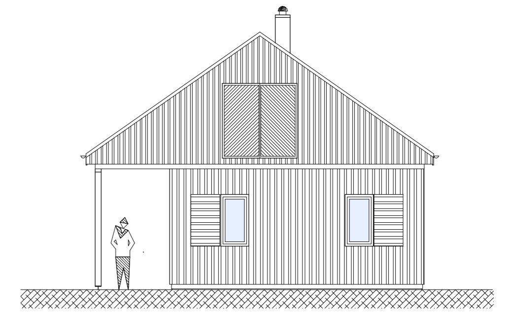
ANSICHT SÜDOSTEN
