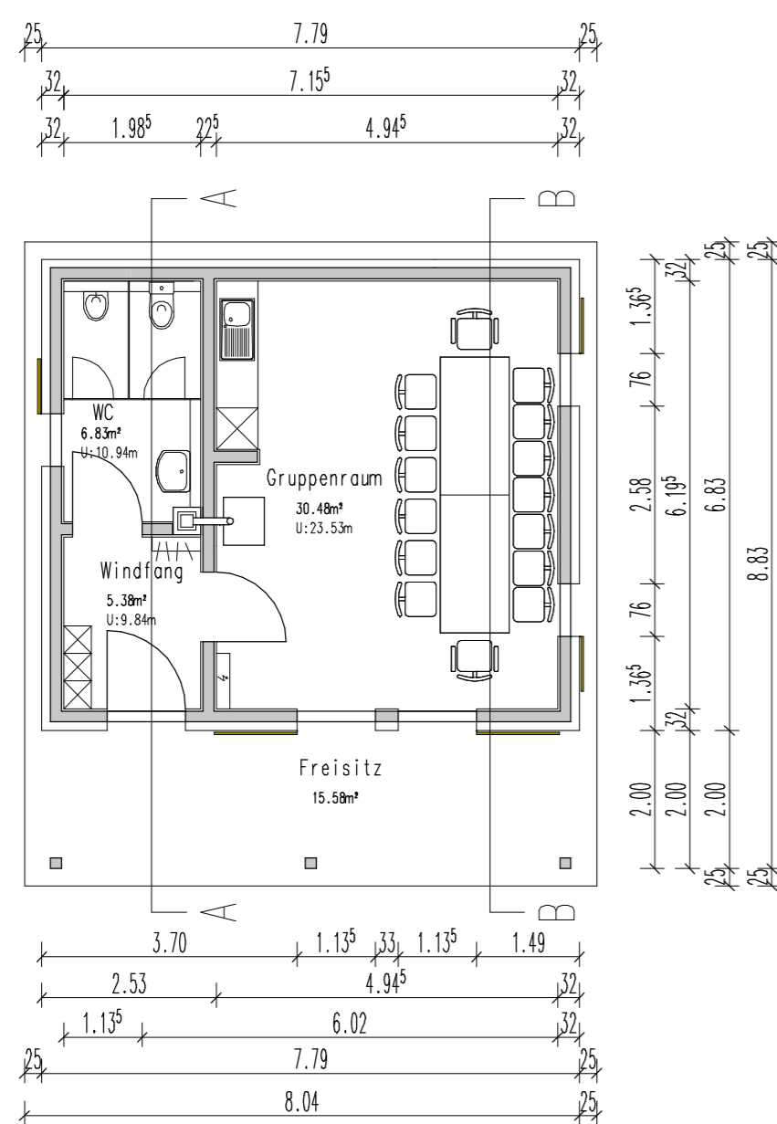
GRUNDRISS ERDGESCHOSS
